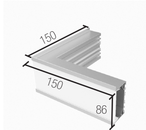
(L*W*H) 150*150*86 mm
