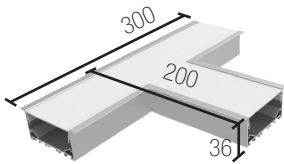
(L*W*H) 300*300*36 mm
