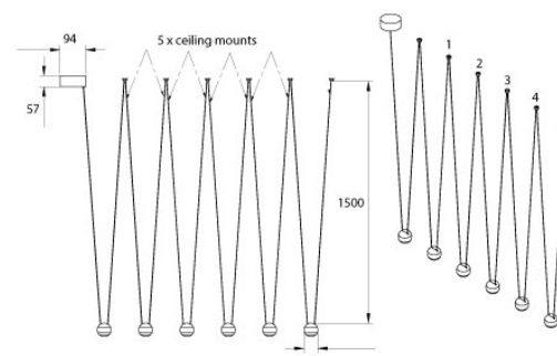
AD-P 77-6 Ø 79 x 1500
