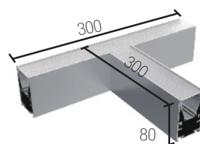
(L*W*H) 300*300*80 mm
