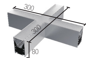
(L*W*H) 300*300*80 mm
